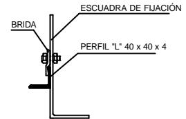
DETALLE B UNIÓN PERFIL-ESCUADRA
